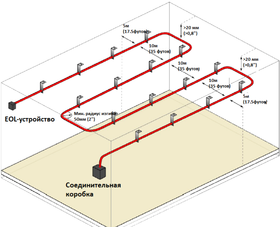
Изображение 10: Защита больших площадей при помощи Термокабеля LHD* *При проектировании и монтаже термокабеля необходимо ориентироваться на внутри Российские нормативные документы.
